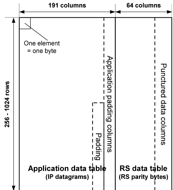
Fig. 6. MPE-FEC frame.
